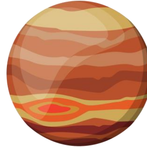
Jupiter
