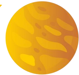
Venus
